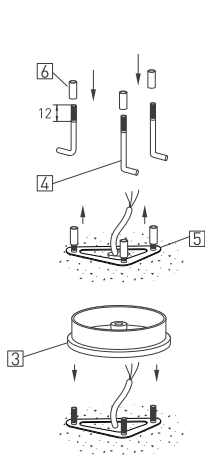
Рис. 3. Установка и подключение светильника
