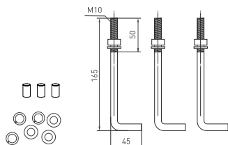
Рис. 2. Чертеж элементов закладной части светильника
