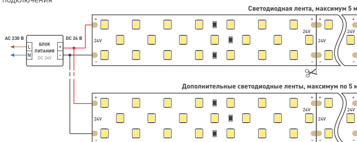
Схема 1. Подключение нескольких светодиодных лент с одной стороны
