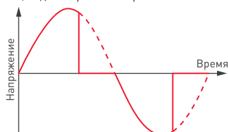
Диммирование с отсечкой заднего фронта.
