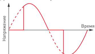
Диммирование с отсечкой переднего фронта.
